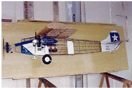
Demi éclaté de l'avion FOKKER F VII « América » Ech : 7 ième
