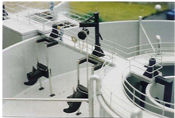
Détails des matériels utilisés dans les bassins biologiques
